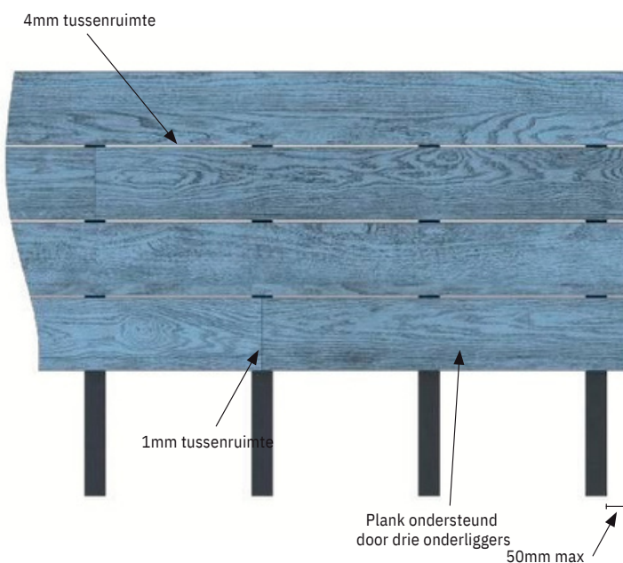
Algemene tussenruimtes
