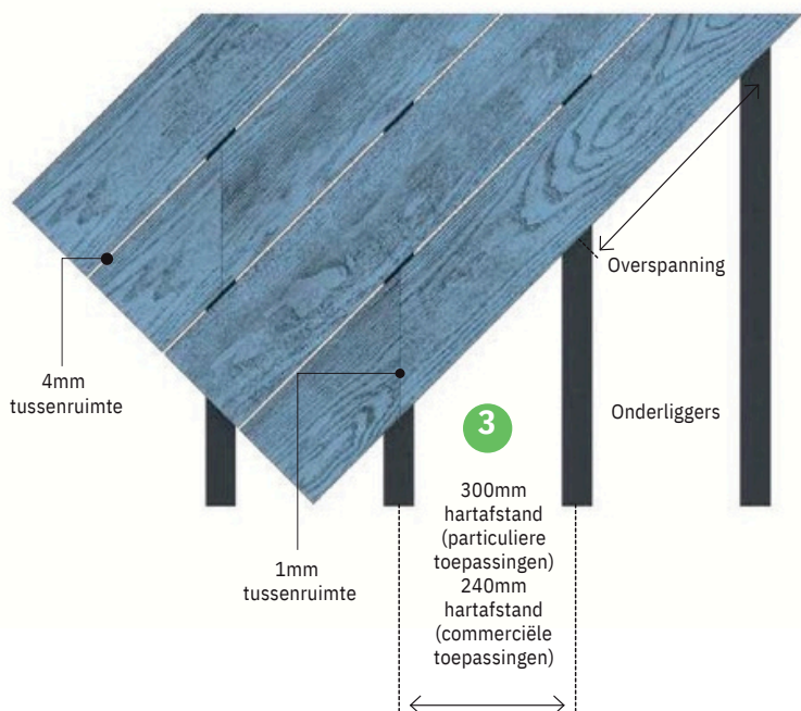
Hartafstanden voor planken op 45°
