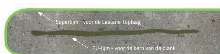
Locatie van de lijm bij verstekhoeken
