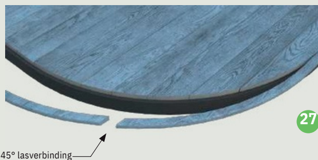
Randafwerkingen verbinden
